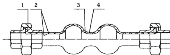
图 5 喉箍连接的可挠橡胶接头结构示意图
