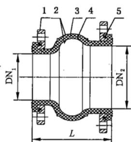
f) 单球体突面法兰密封同心异径 XT Q_1Y_tRF_1^*
